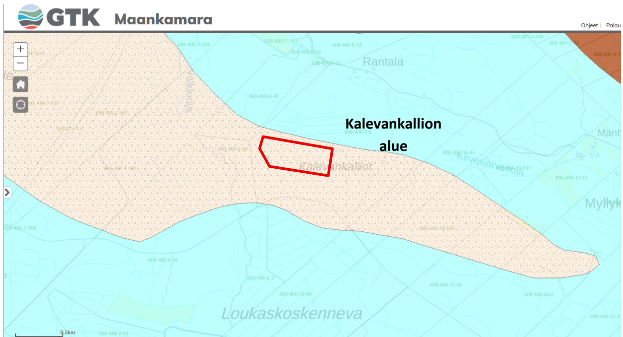
Kuva 2. Kallioperäkartta. Ottamisalue on osoitettu rajauksena. Alueen kallioperä koostuu sekä tonaliitista ja mahdollisesti pohjoisreunassa on kiillegneissiiä/suonigneissiiä. Mittajana 0,2 km on kartan vasemmassa alakulmassa. Lähde: GTK, Maanmittauslaitos, Esri Finland 2026.
