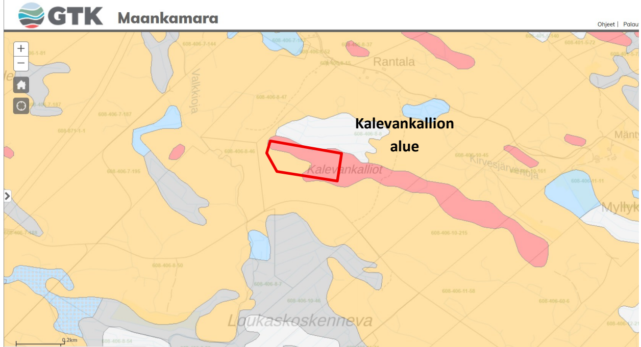
Kuva 1. Maaperäkartta. Ottamisalue on osoitettu rajauksena. Alueen pintamaalajina on hienoainesmoreenia (HMr) ja paljalla alueilla kalliomaata Ka (punainen). Pohjamaalaji on kaikkialla kalliomaata. Pohjoispuolella on pienialaisesti rahkaturvetta St (valkoinen). Mittajana 0,2 km on kartan vasemmassa alakulmassa. Lähde: GTK, Maanmittauslaitos, Esri Finland. 2026.
